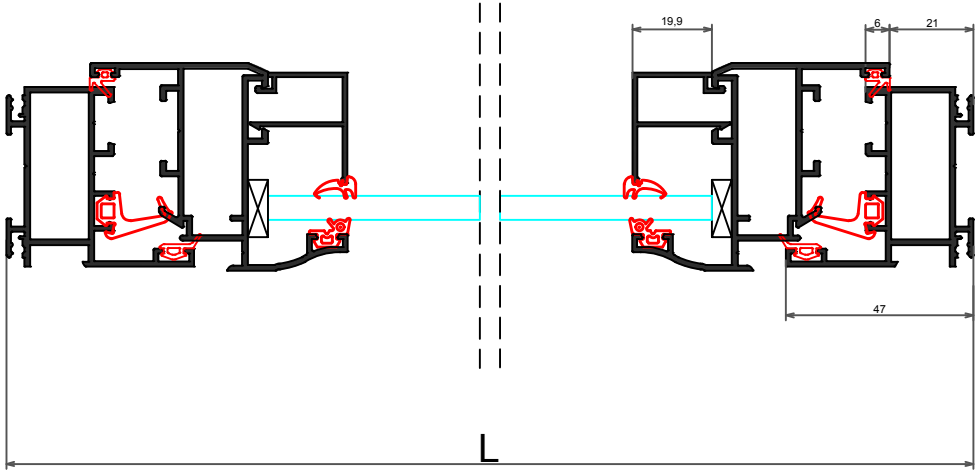
COUPE B-B
