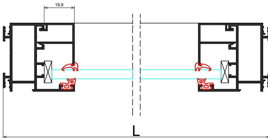
COUPE B-B
