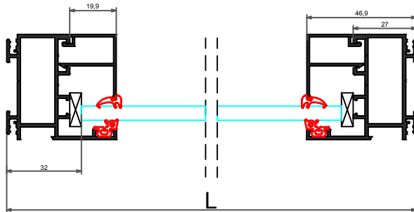
COUPE C-C
