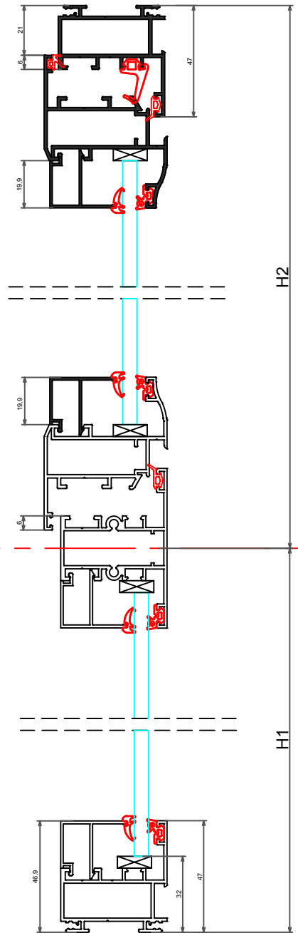
COUPE A-A
