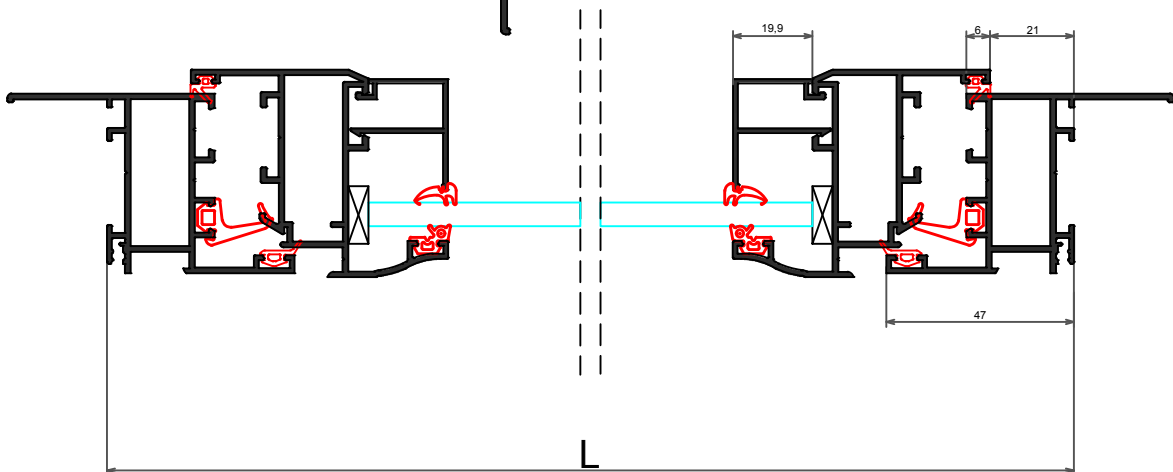
COUPE B-B
