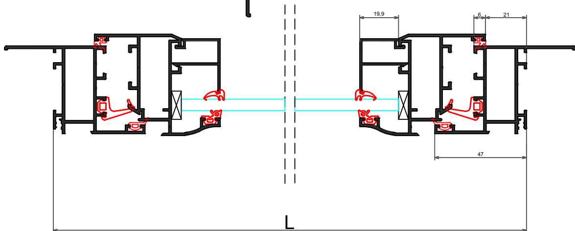
COUPE B-B
