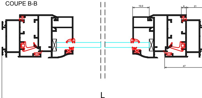
COUPE B-B
