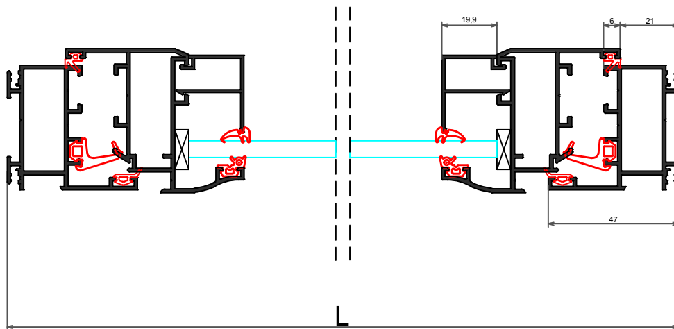
COUPE B-B
